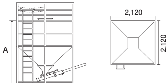
鋼板製屋内燃料タンク仕様表 ※現場に合わせての特注となります。(安全柵・ハンゴ付)
